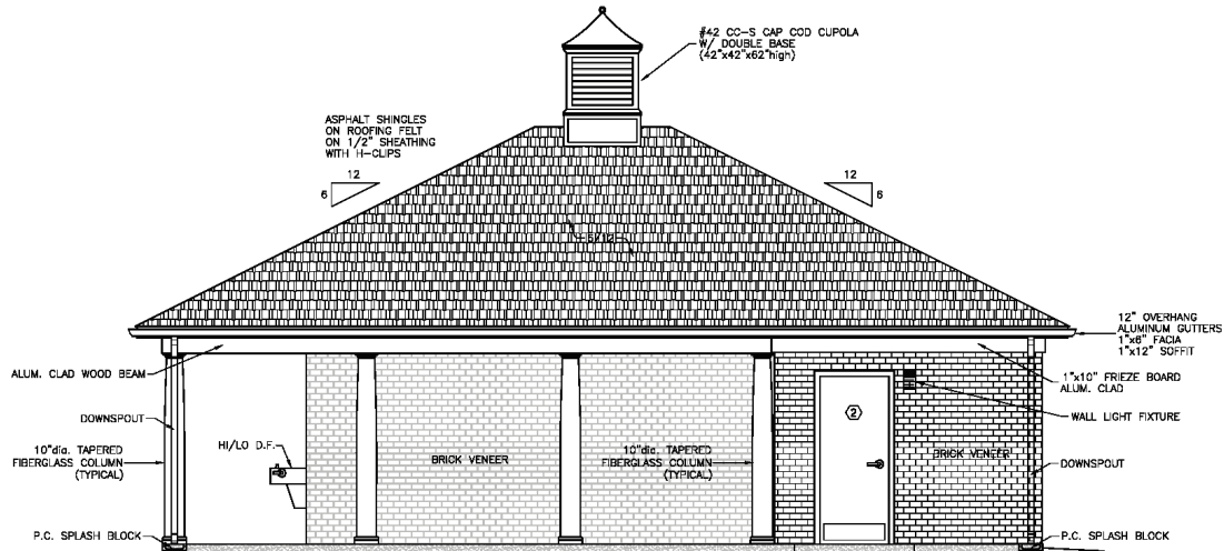
Right Elevation
