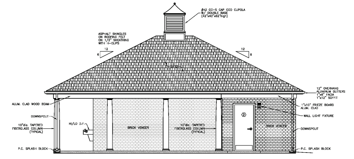
Right Elevation
